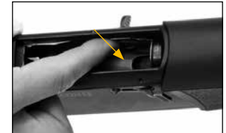
Нажмите внутрь на упор для разряжания магазина
